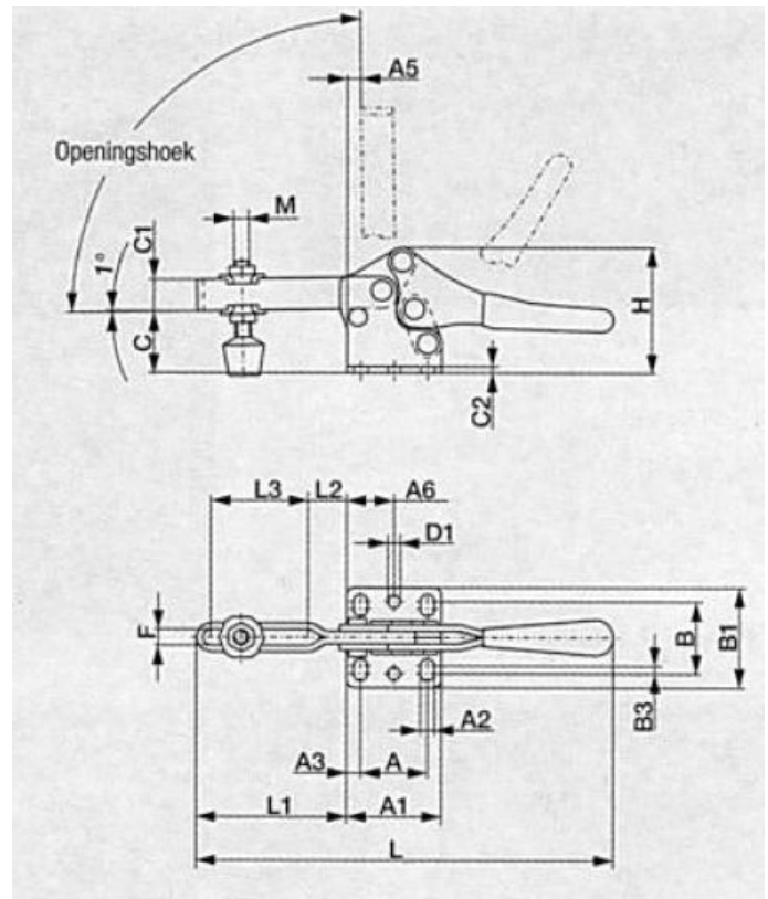
bovenaanzicht
